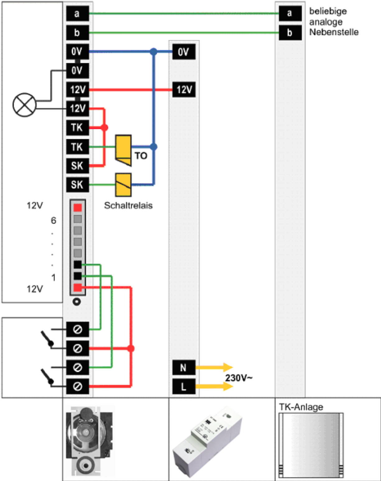
Anschaltung des ET400-ab
