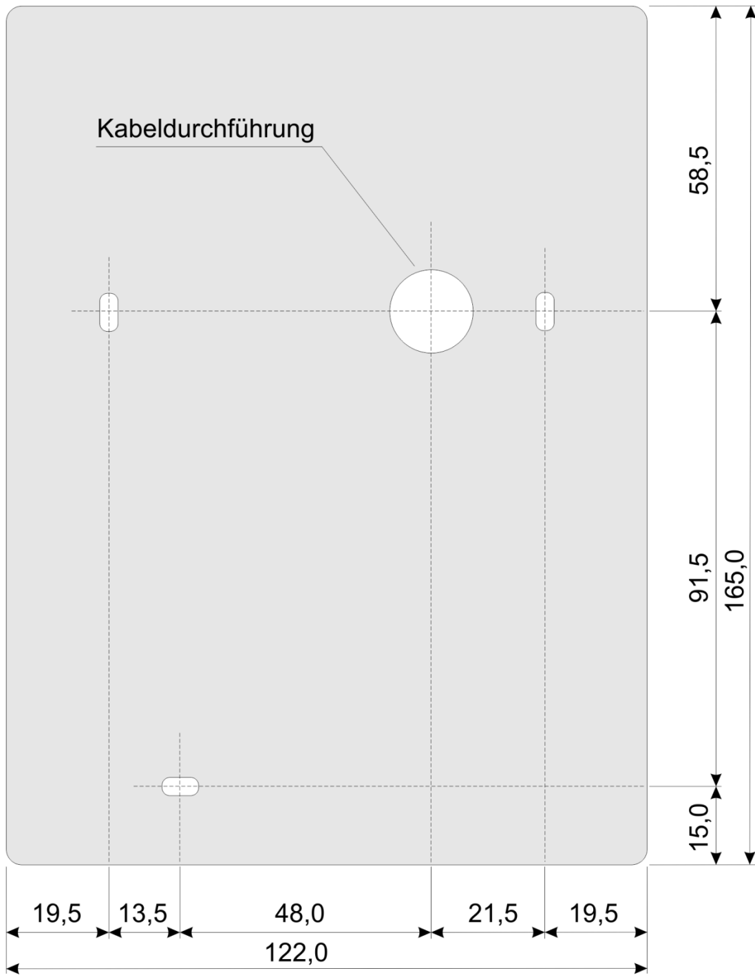
Gehäuseabmessungen der Keil doorTEL GSM Rev 2 (Draufsicht, nicht maßstabsgerecht)
